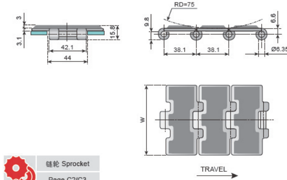
SS812/815G 防滑单铰直输平顶链 SS812/815G WITH RUBBER TOP
