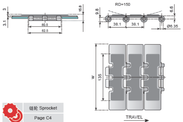
SS802/805G 防滑双铰直输平顶链 SS802/805G WITH RUBBER TOP
